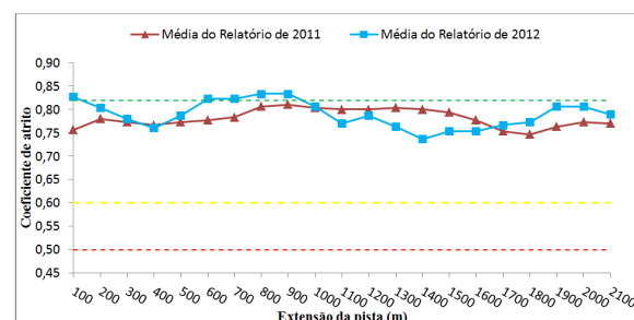
Figura 8: Gráfico do coeficiente de atrito a 3 metros do eixo da pista de pouso e decolagem, em 2011 e 2012.
