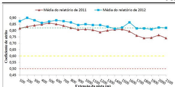
Figura 9: Gráfico do coeficiente de atrito a 6 metros do eixo da pista de pouso e decolagem, em 2011 e 2012.
