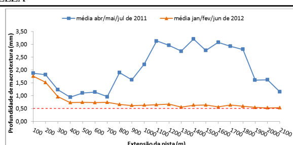
Figura 3: Gráfico da profundidade média da mancha de areia na pista de pouso e decolagem, em 2011 e 2012.
