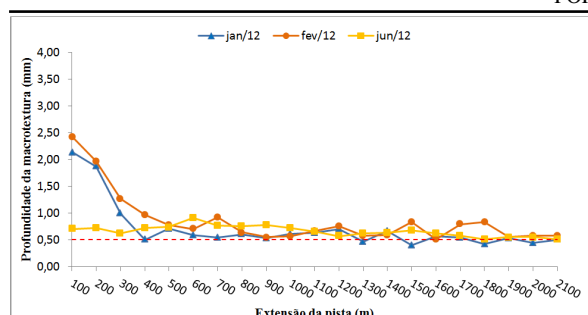
Figura 2: Gráfico da profundidade média da mancha de areia na pista de pouso e decolagem, em 2012.
