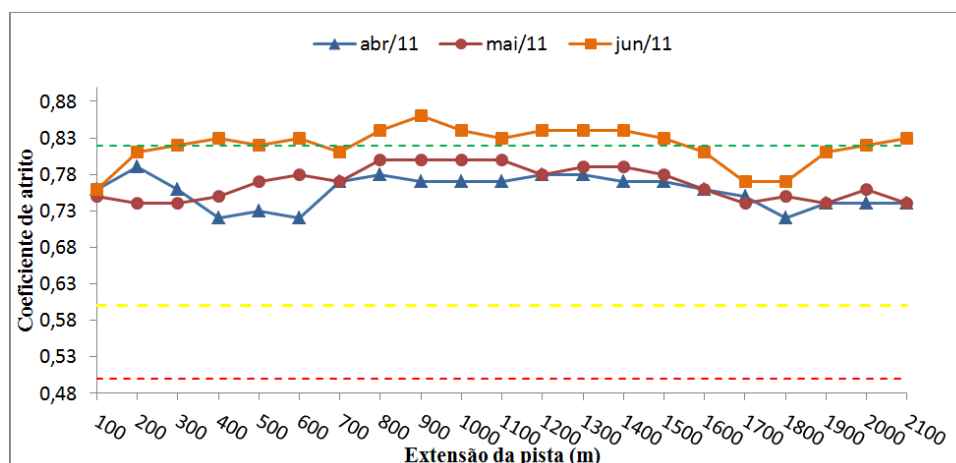
Figura 4: Gráfico do coeficiente de atrito a 3 metros do eixo da pista de pouso e decolagem, em 2011.
