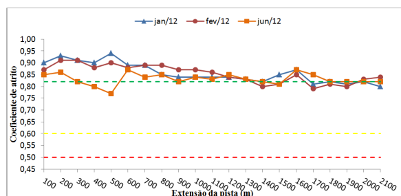
Figura 7: Gráfico do coeficiente de atrito a 6 metros do eixo da pista de pouso e decolagem, em 2012.
