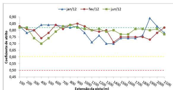
Figura 6: Gráfico do coeficiente de atrito a 3 metros do eixo da pista de pouso e decolagem, em 2012.
