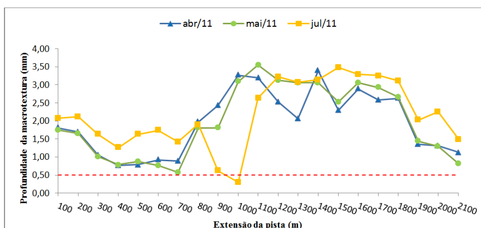
Figura 1: Gráfico da profundidade média da mancha de areia na pista de pousos e decolagens, em 2011.
