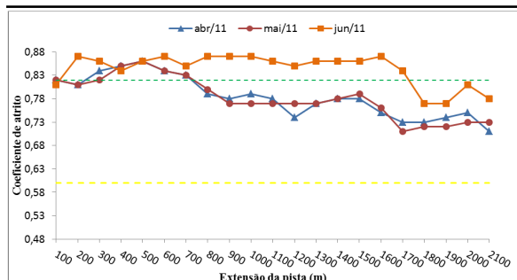
Figura 5: Gráfico do coeficiente de atrito a 6 metros do eixo da pista de pouso e decolagem, em 2011.
